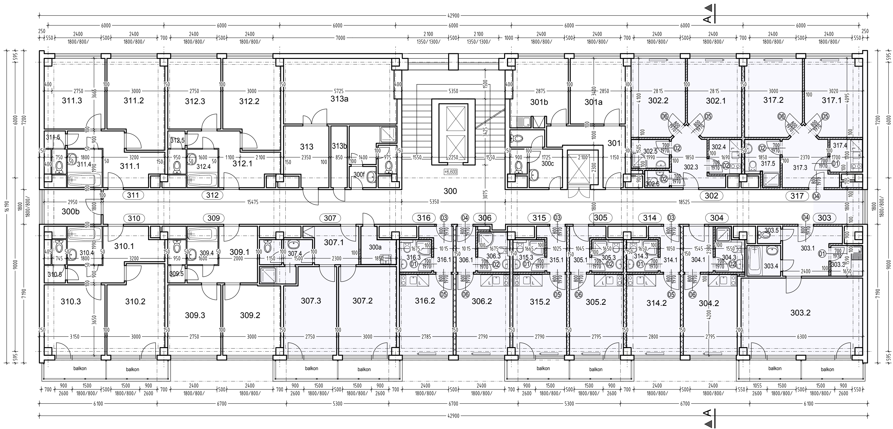
TABULKA MÍSTNOSTÍ 2.P = 3.NP
