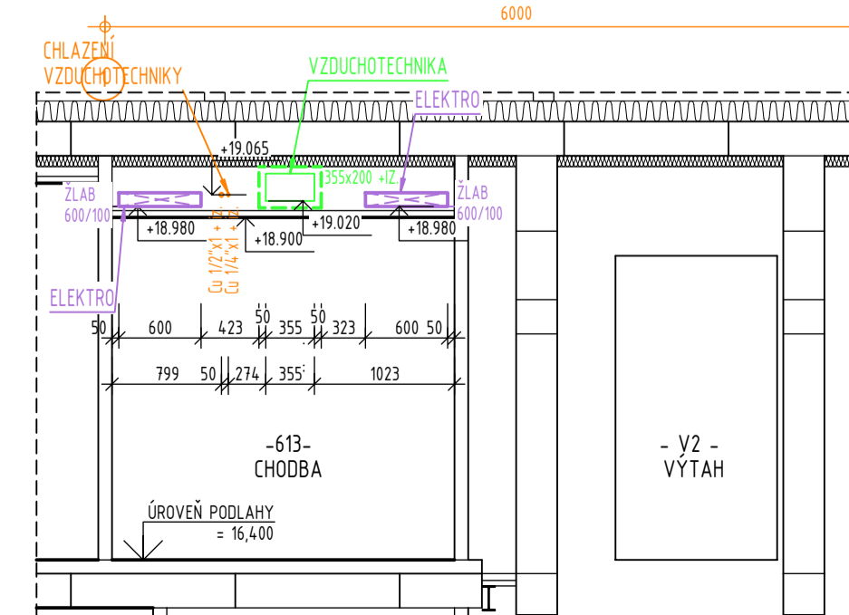
KOORDINAČNÍ ŘEZ K2 M 1 : 50
