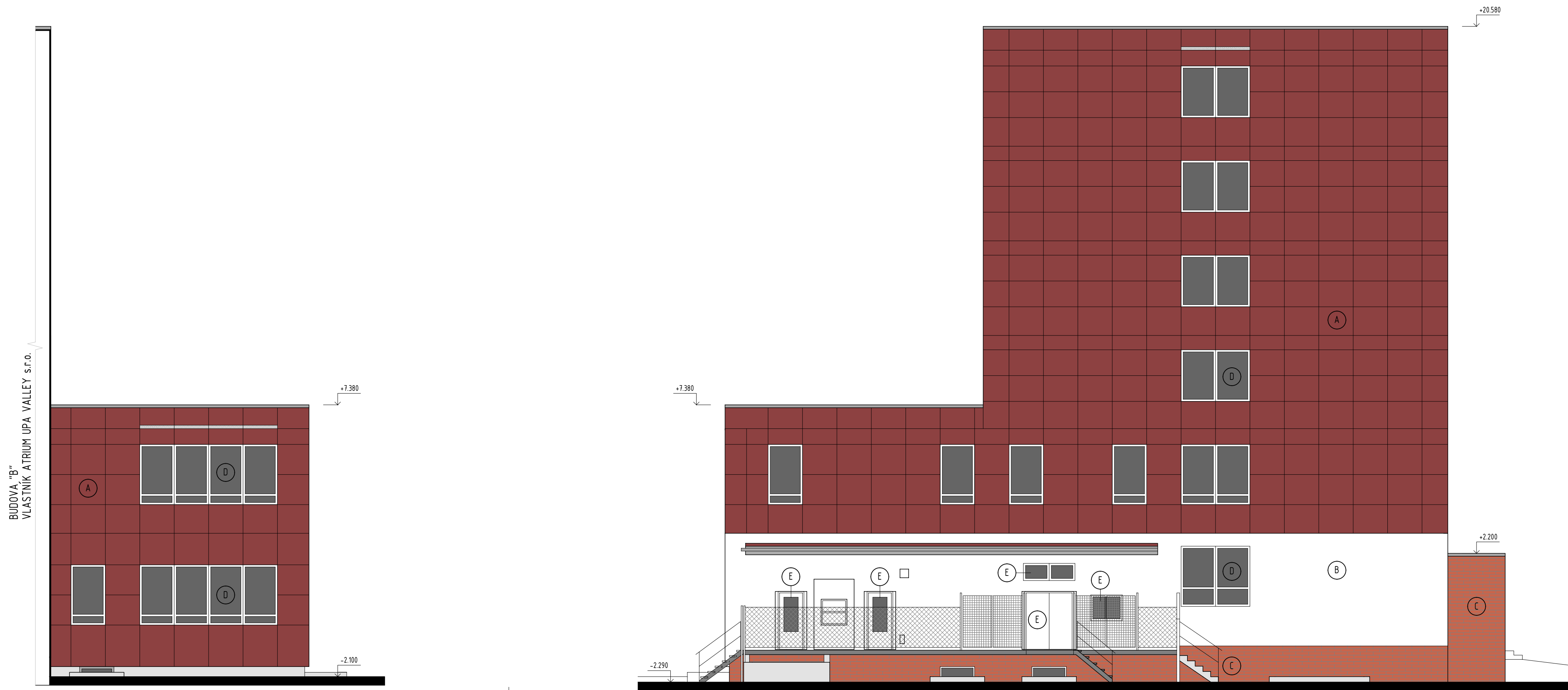
POHLED JIHOVÝCHODNÍ - STÁVAJÍCÍ STAV, M 1:100
